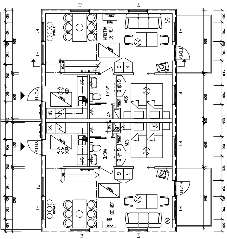
ÖVRE PLAN
