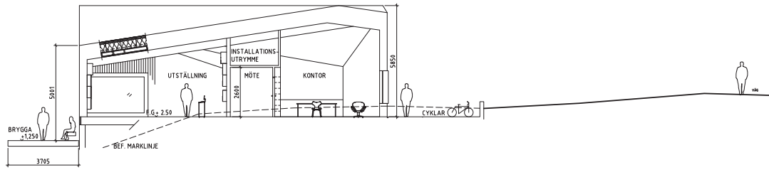
SEKTION B-B
